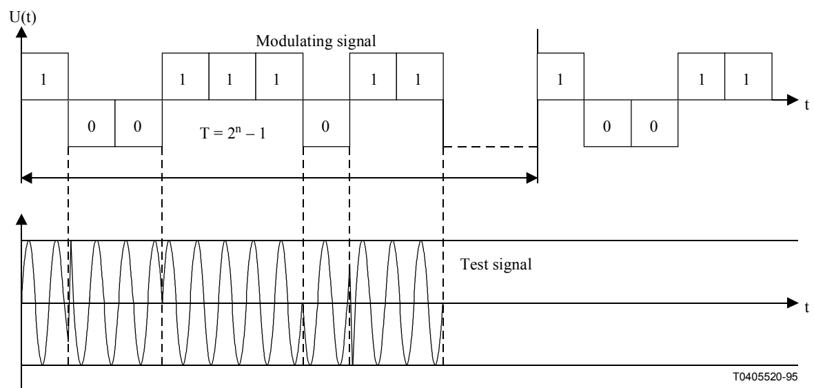
Figura I.3/O.1 – Señal moduladora y señal de prueba
