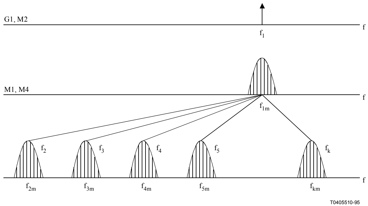
Figura I.2/O.1 – Diagrama de frecuencias del aparato de medida de la diafonía
