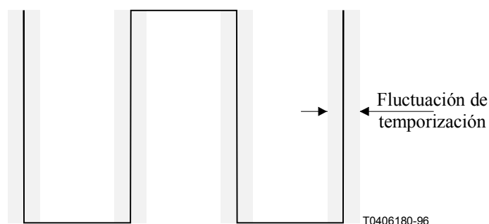
Figura 3/O.1 – Variación de los cruces por cero que representan la fluctuación de fase de la temporización
