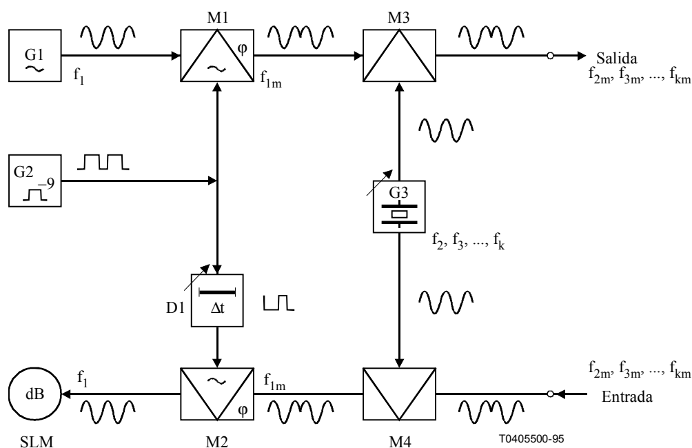
Figura I.1/O.1 – Diagrama de bloques simplificado del aparato de medida de la diafonía
