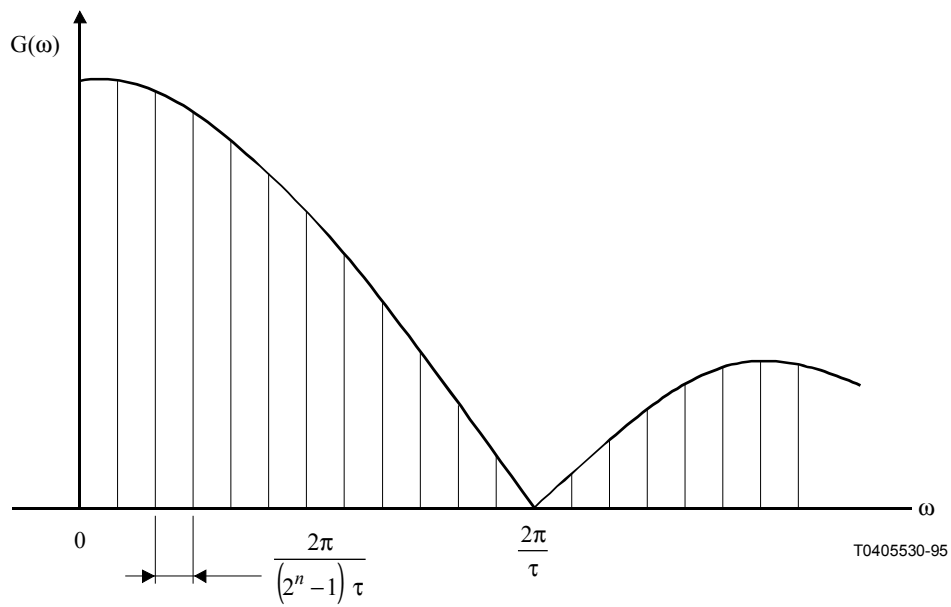
Figura I.4/O.1 – Espectro de la señal moduladora
