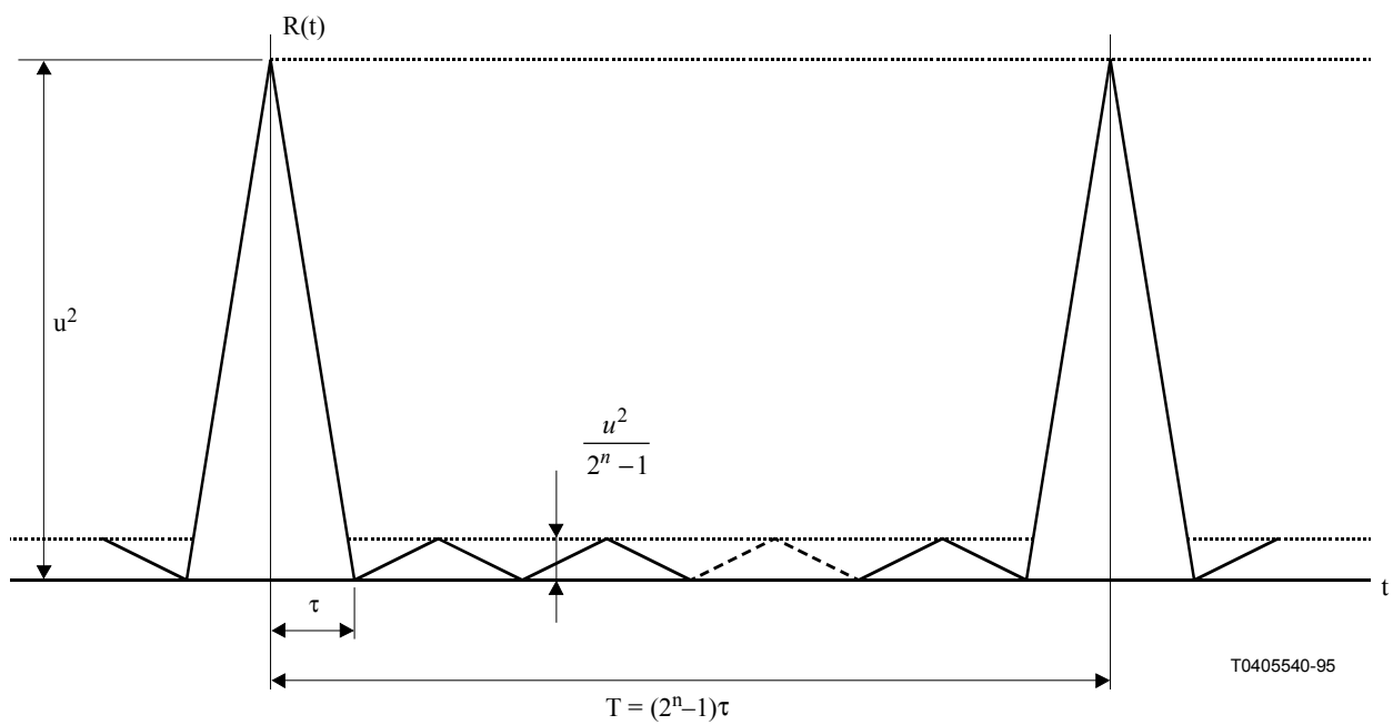
Figura I.5/O.1 – Función de correlación de la señal de prueba
