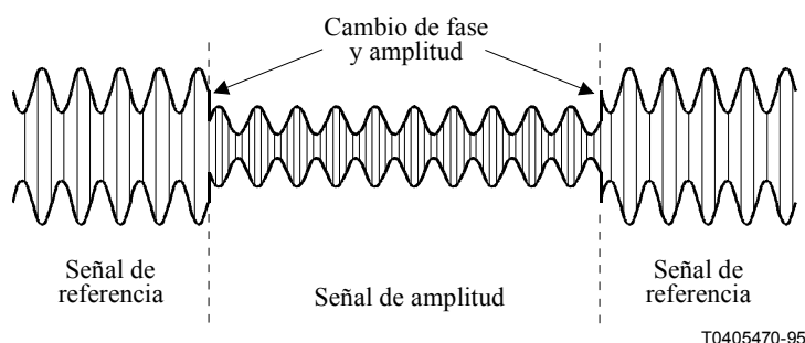
Figura 1/O.1 – Señal de prueba para la medición de la distorsión de retardo de grupo y de amplitud
